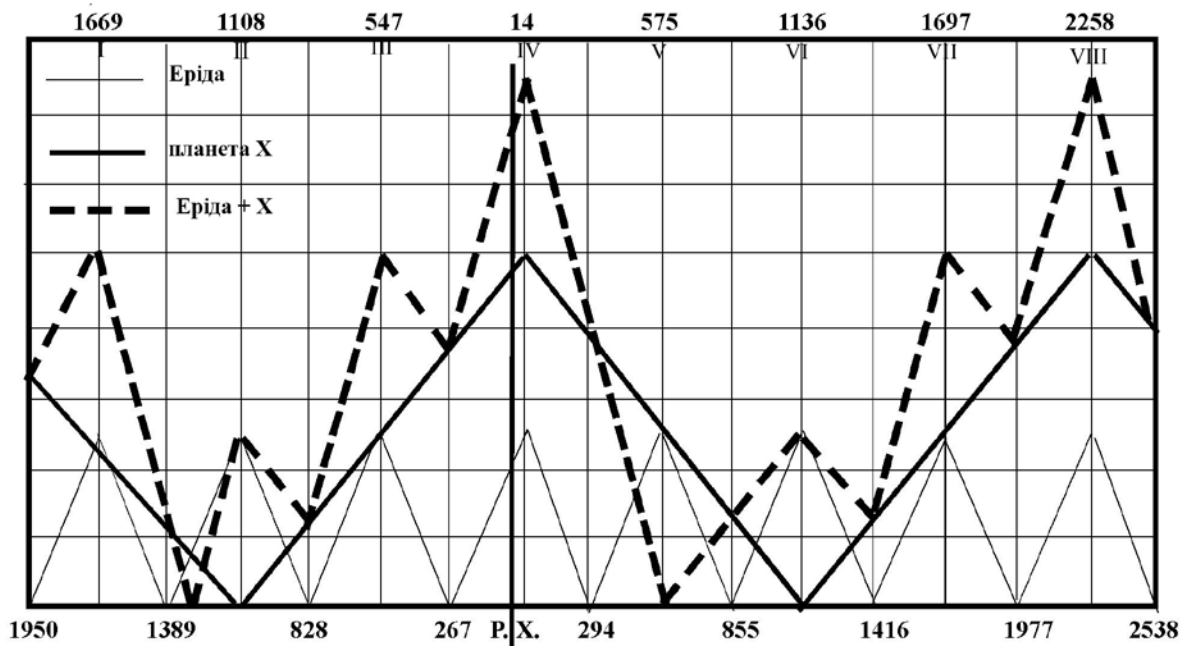
Рис. 1. Пунктиром показано сумарну амплітуду коливань Ериди та планети X, якщо амплітуда коливань планети X буде вдвічі більшою ніж у Ериди.
