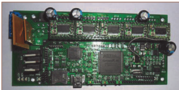
Розроблений модуль на базі Altera Cyclone III EP3C10E144I7N
