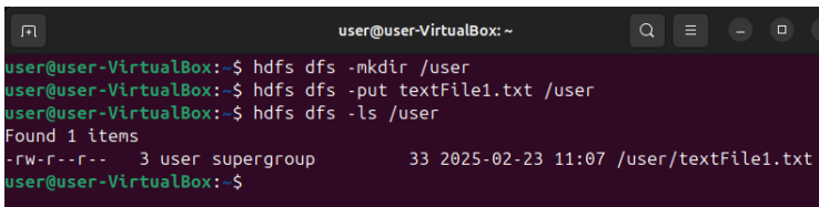
Мал. 48 – Створення каталогу, завантаження файлу та перегляд вмісту HDFS
