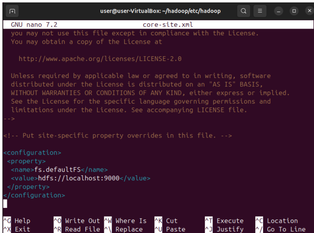
Мал. 38 – Редагування конфігураційного файлу core-site.xml
