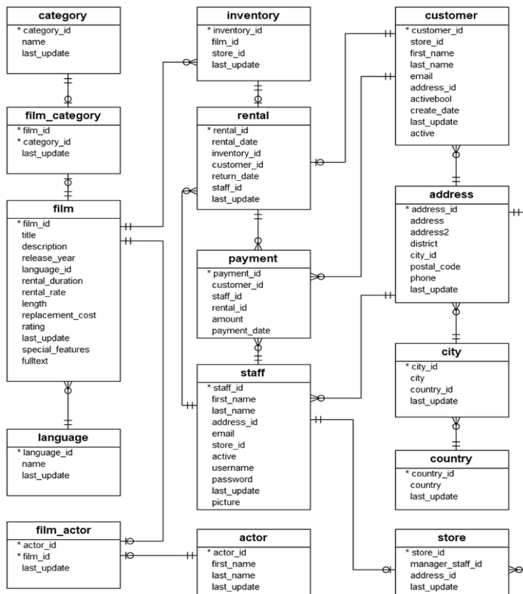
Мал. 1 – Схема бази даних Pagila
