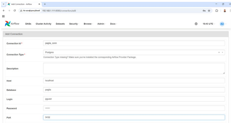
Мал. 32 – Заповнення параметрів підключення PostgreSQL в Apache Airflow
