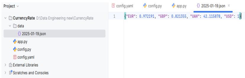
Мал. 9 – Структура проєкту та приклад JSON-файлу з отриманими курсами валют
