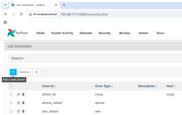
Мал. 31 – Створення нового підключення PostgreSQL у вебінтерфейсі Airflow
