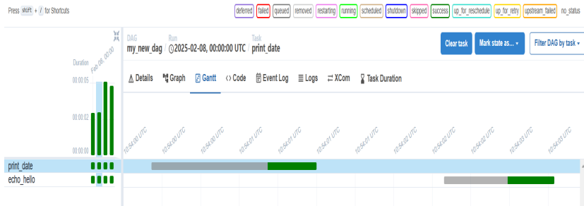
Мал. 27 – Відображення тривалості виконання завдань у режимі Gantt Chart
