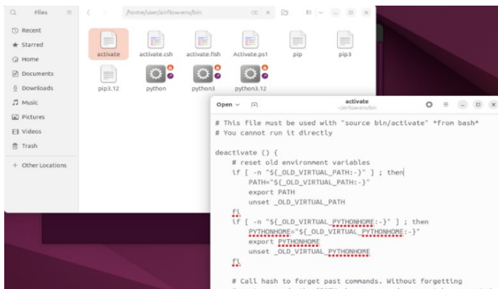
Мал. 11 – Вміст bash -скрипта activate для активації віртуального середовища
