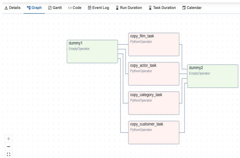
Мал. 33 – Граф DAG для експорту таблиць із бази даних PostgreSQL
