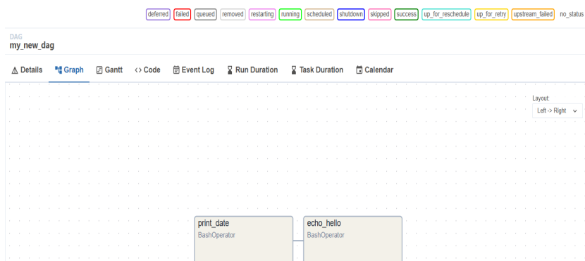
Мал. 25 – Графічне представлення структури DAG у режимі Graph View
